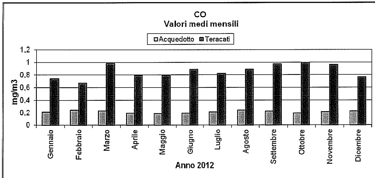
Grafico 13 : CO medie mensili
