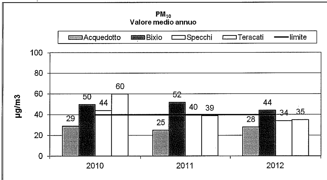
Grafico 18 : PM10: Valore medio annuale
