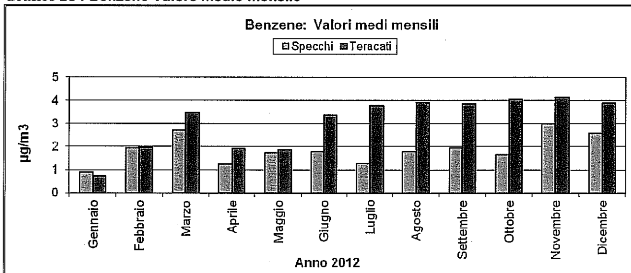
Grafico 21 : Benzene Valore medio mensile
