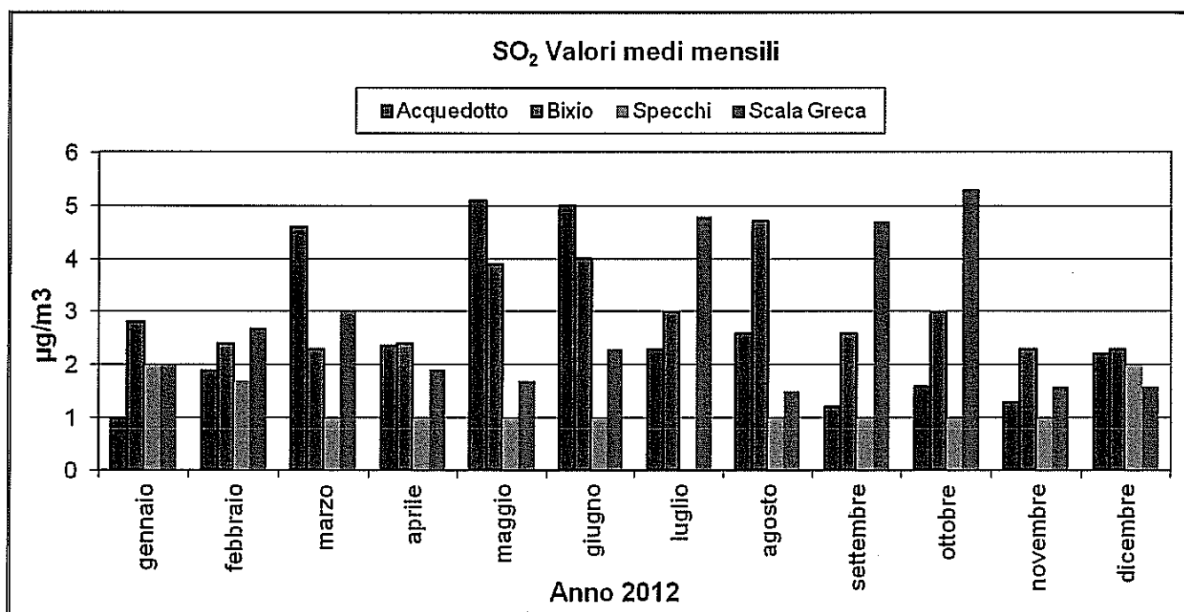
Grafico 7 : SO 2 valori medi mensili
