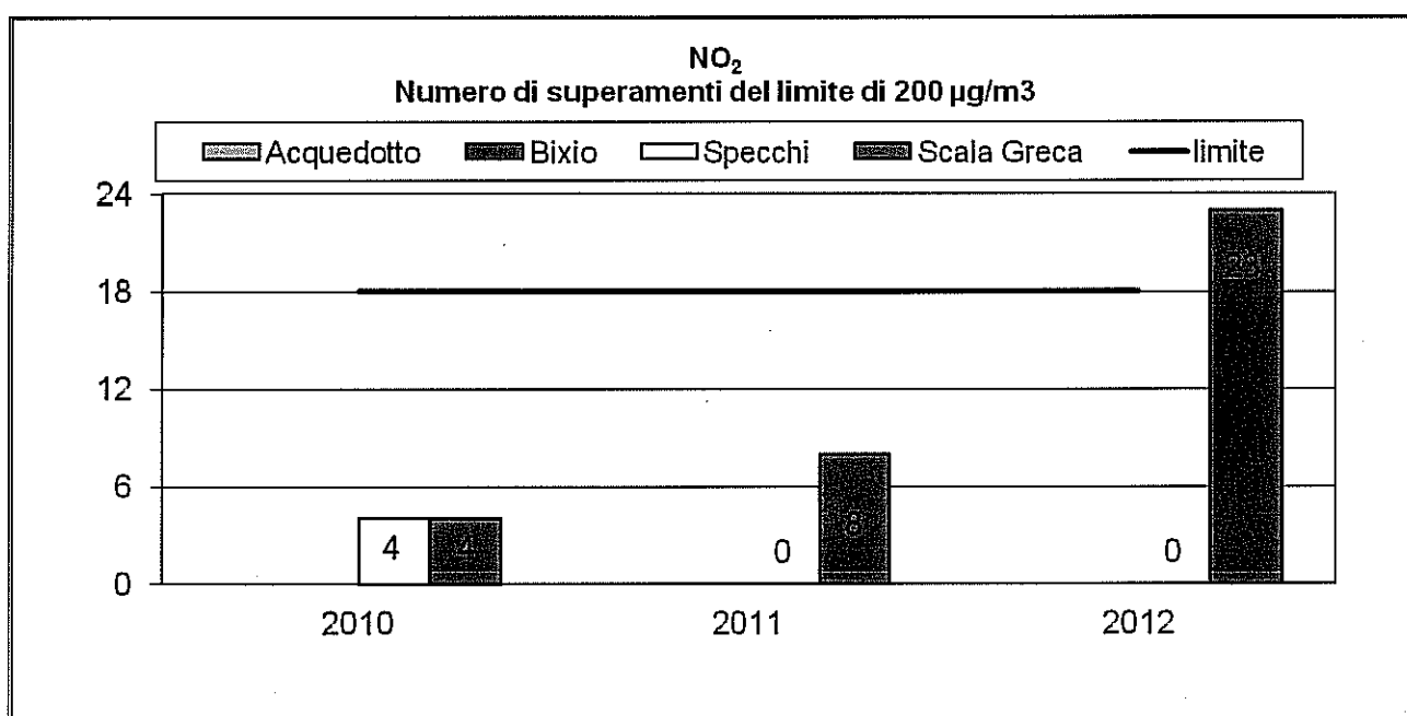
Grafico 8 : NO 2 Numero superamenti del limite orario
