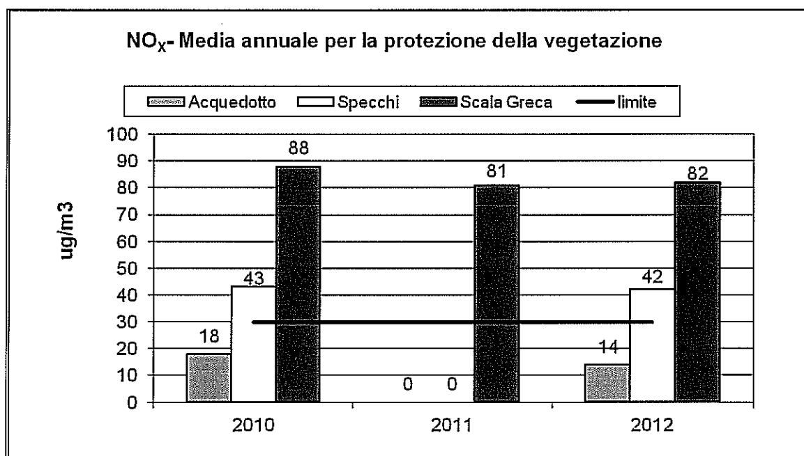
Grafico 11 : NO x : Valore limite annuale per la protezione della vegetazione
