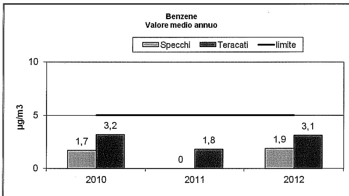
Grafico 20 : Benzene Valore medio annuale
