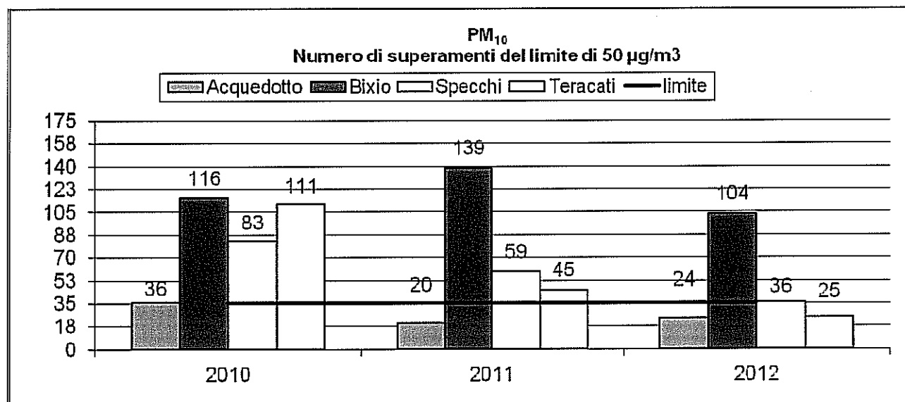
Grafico 17 : PM 10 numero superamenti del limite orario
