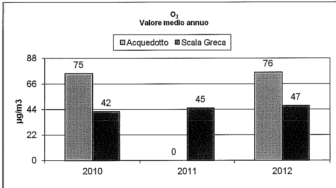
Grafico 15 : O 3 Valore medio annuale
