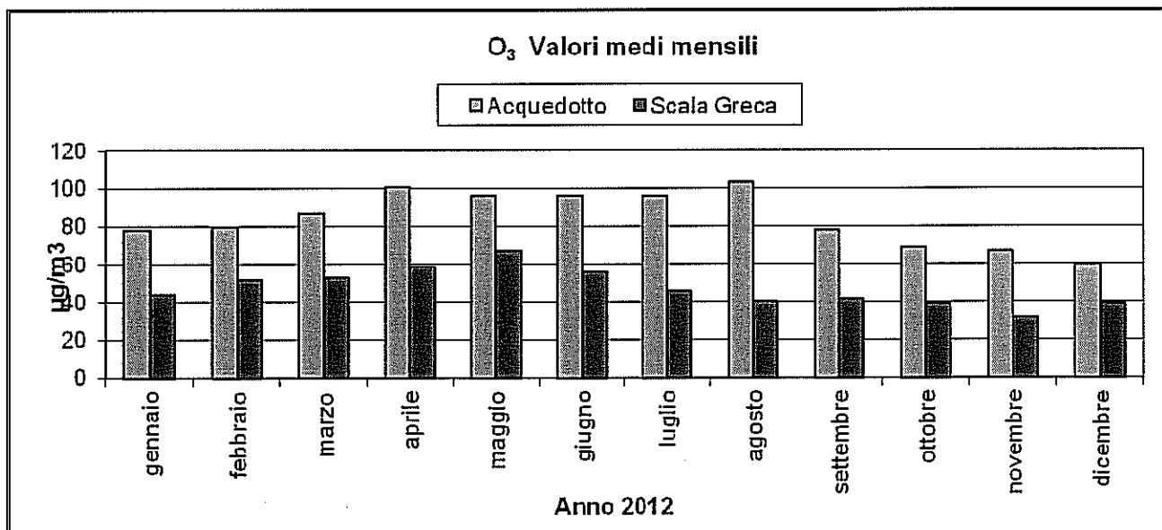
Grafico 16 : O 3 Valori medi mensili
