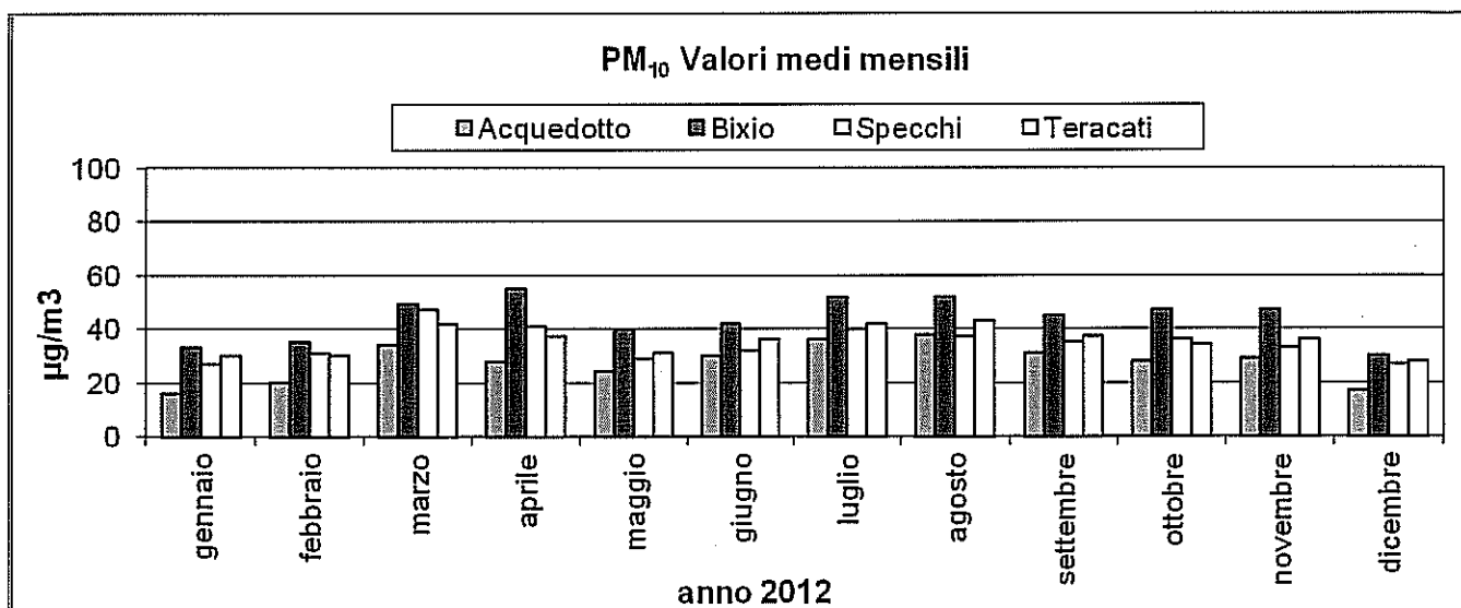
Grafico 19 : PM10 Valore medio mensile
