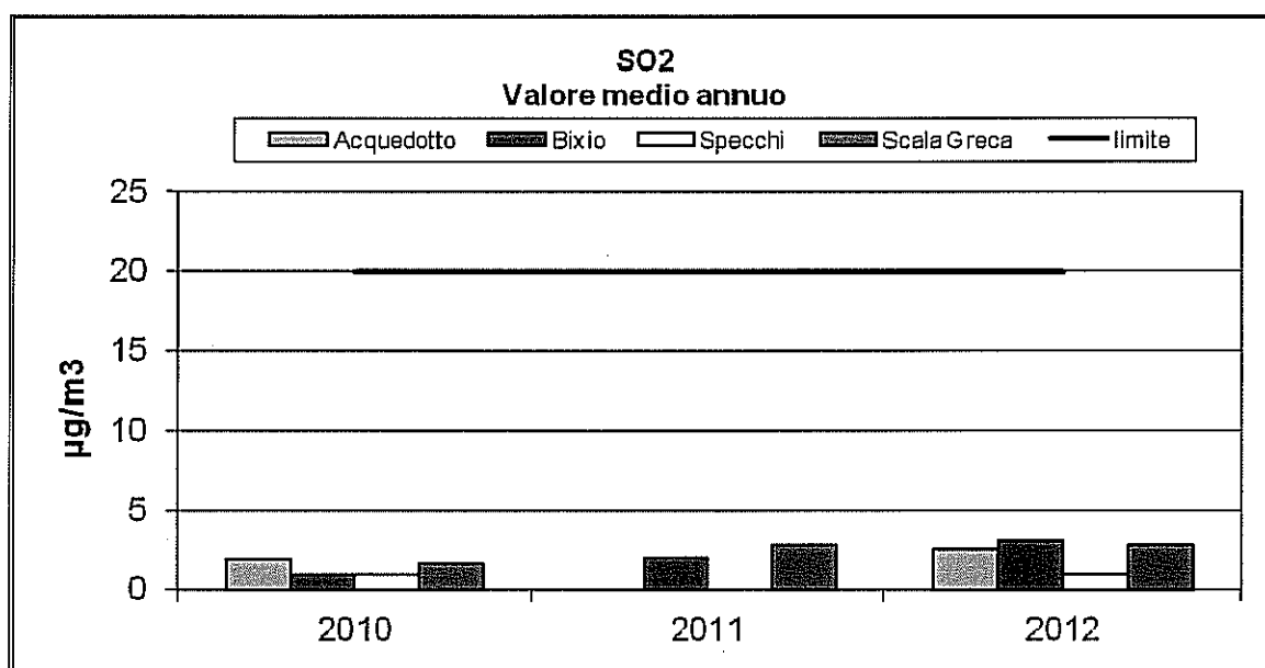
Grafico 6 : SO 2 valori medio annuale
