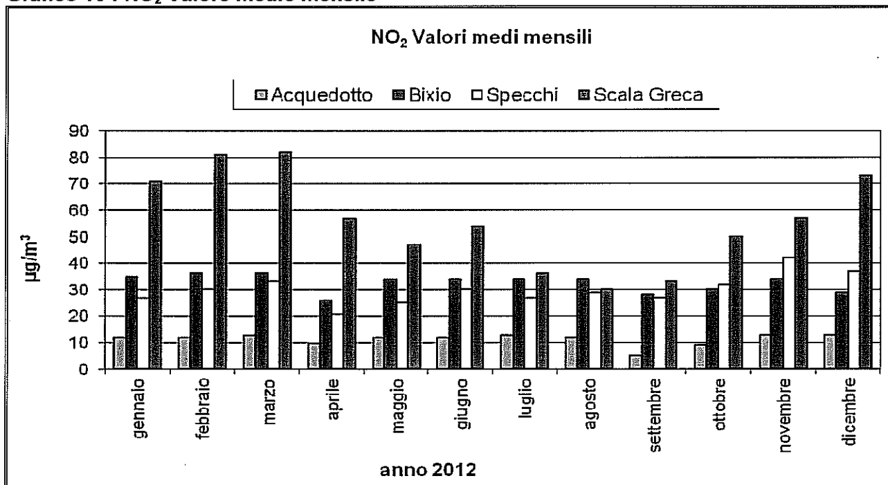
Grafico 10 : NO 2 Valore medio mensile
