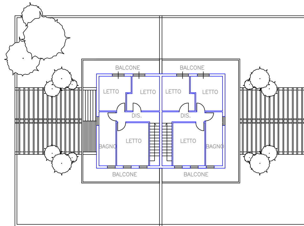
PIANTE PIANO PRIMO SC. 1: 200
