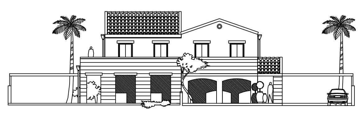
PROSPETTI FRONTE E RETRO SC. 1: 200
