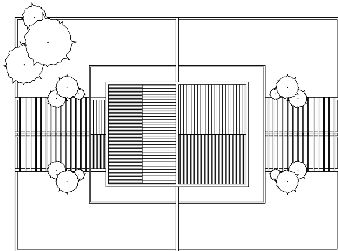
PIANTE PIANO COPERTURE SC. 1: 200
