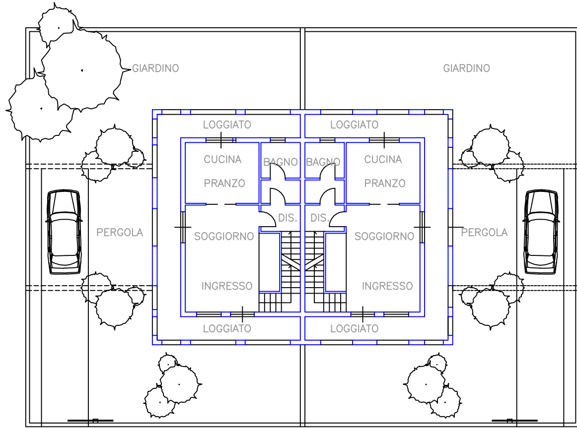
PIANTE PIANO TERRA SC. 1: 200
