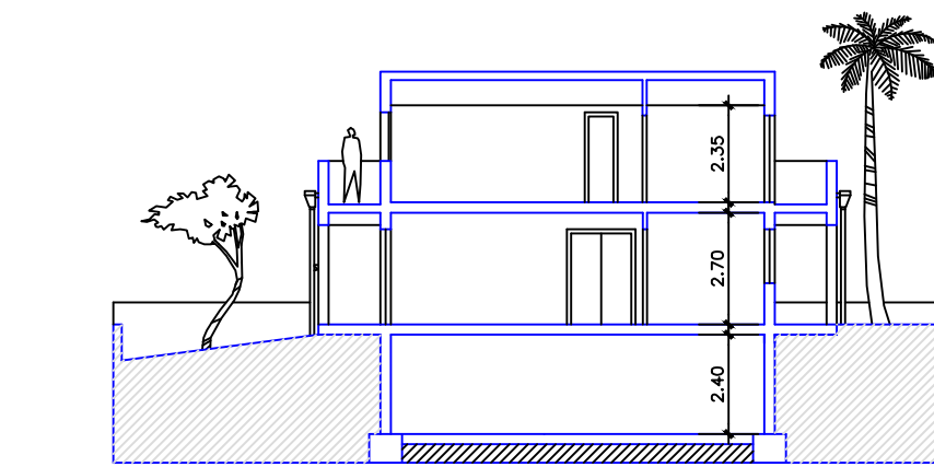
SEZIONE TRASVERSALE SC. 1: 200
